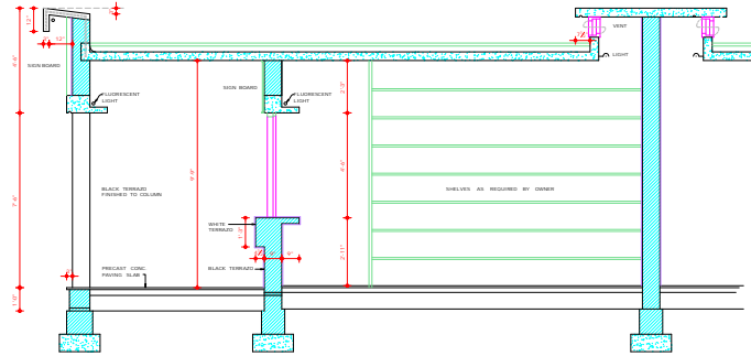
LONGITUDINAL SECTION
